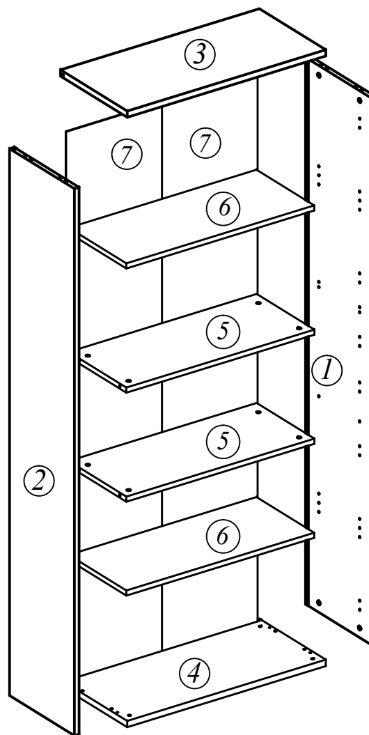
CT-1 (ST-1) - 770x365x1975 CY-1 (SU-1) - 406x365x1975
